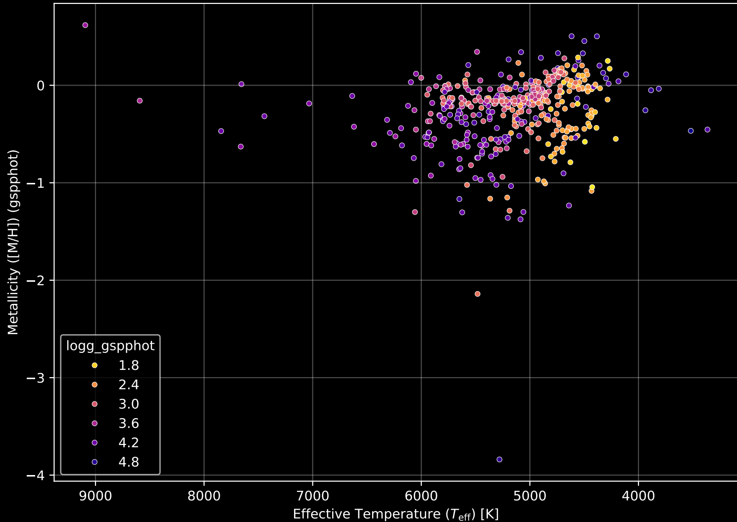
APOGEE DR17 Field: [N2808] Stellar Population Parameters (n= 476)
